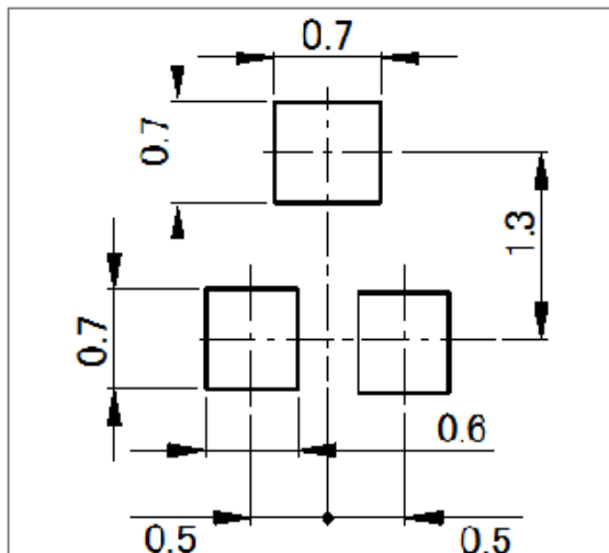
Unit : mm
