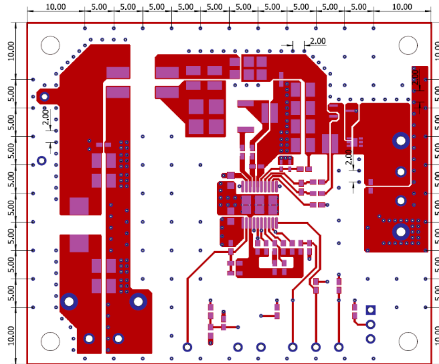
Top layer layout(Top view)
