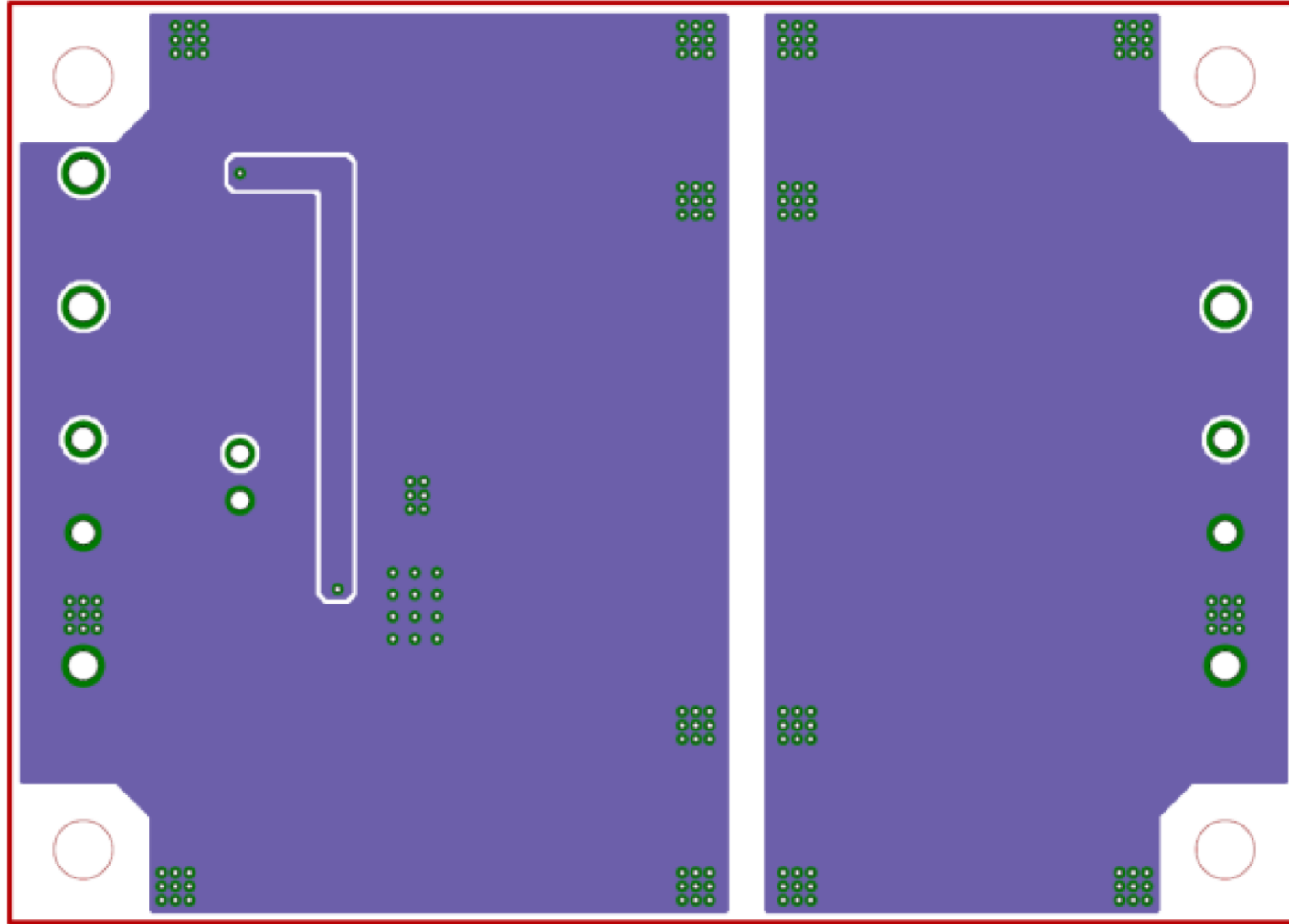
Bottom Side Layer Layout
