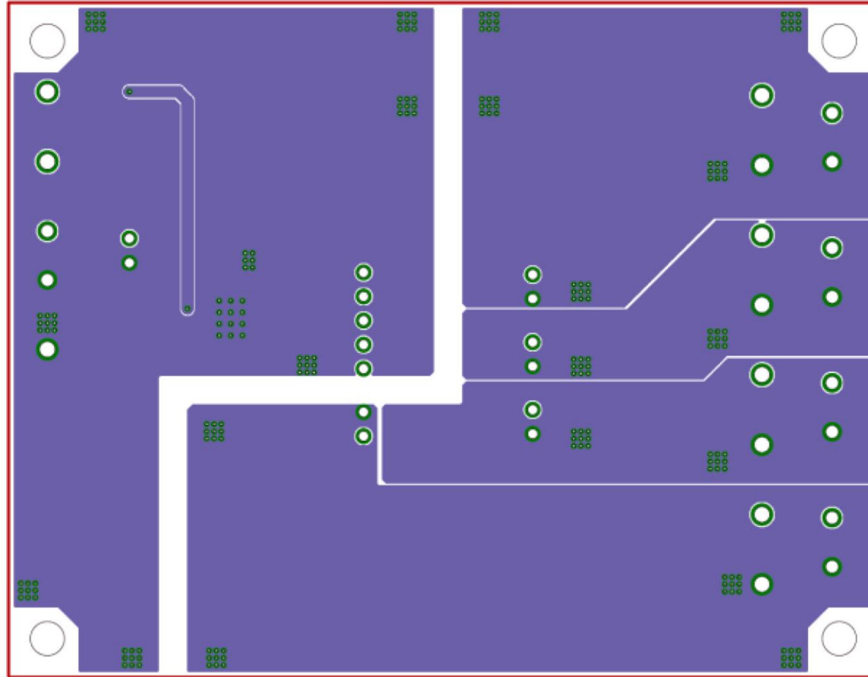
Bottom Side Layer Layout
