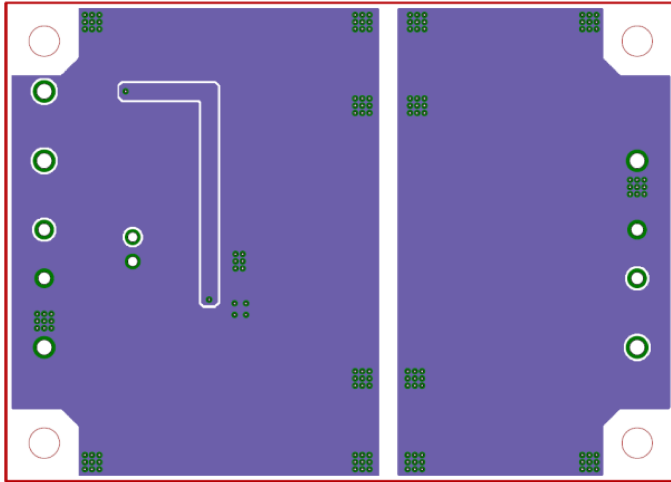
Bottom Side Layer Layout
