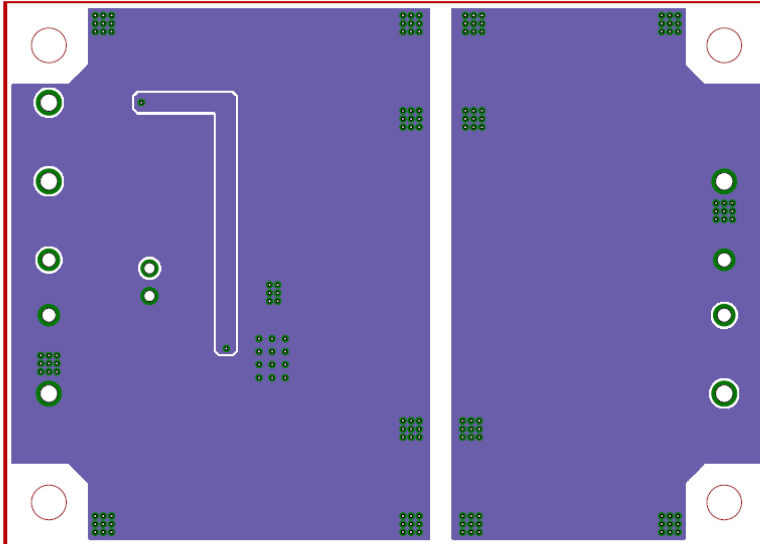
Bottom Side Layer Layout
