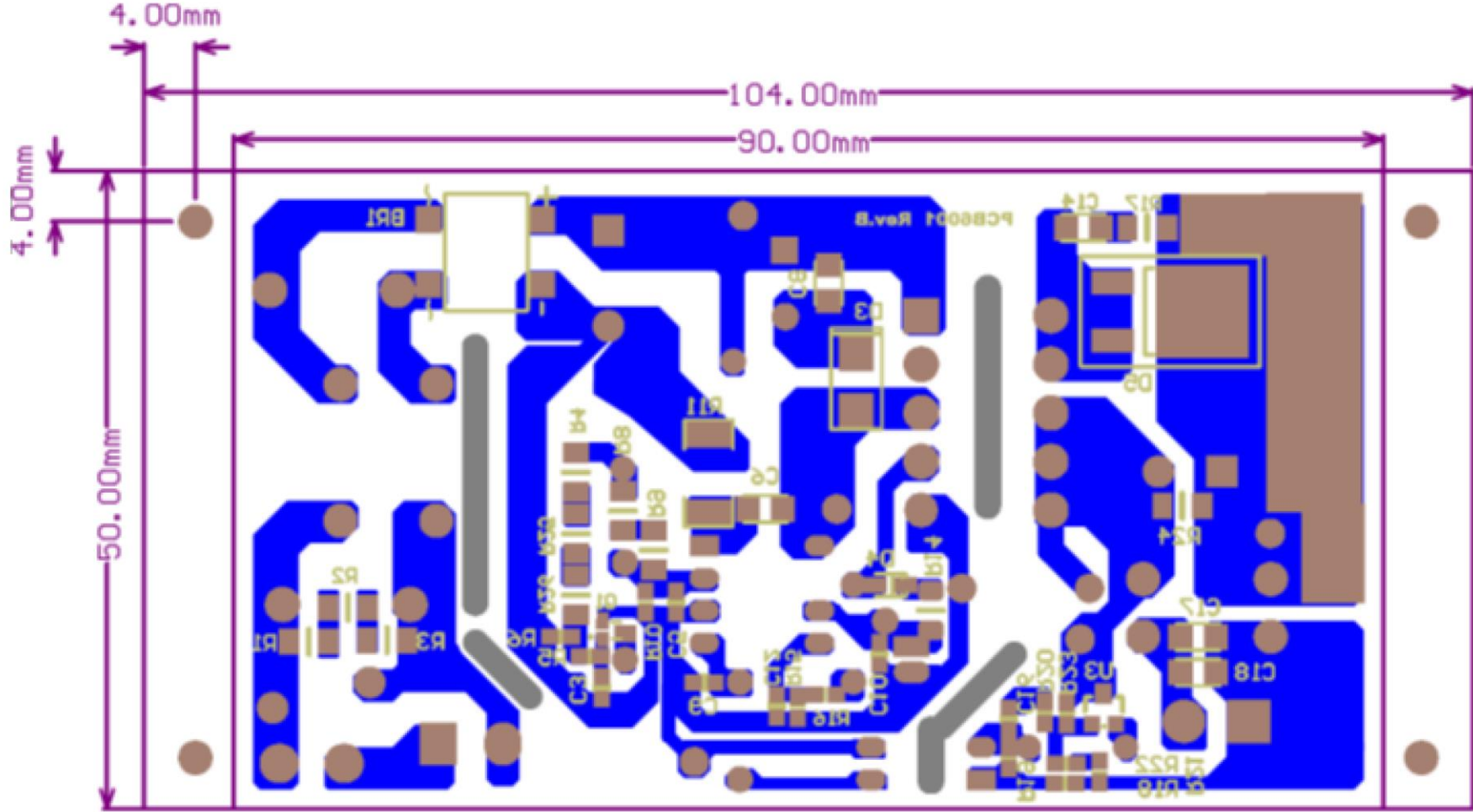
Bottom Layer
