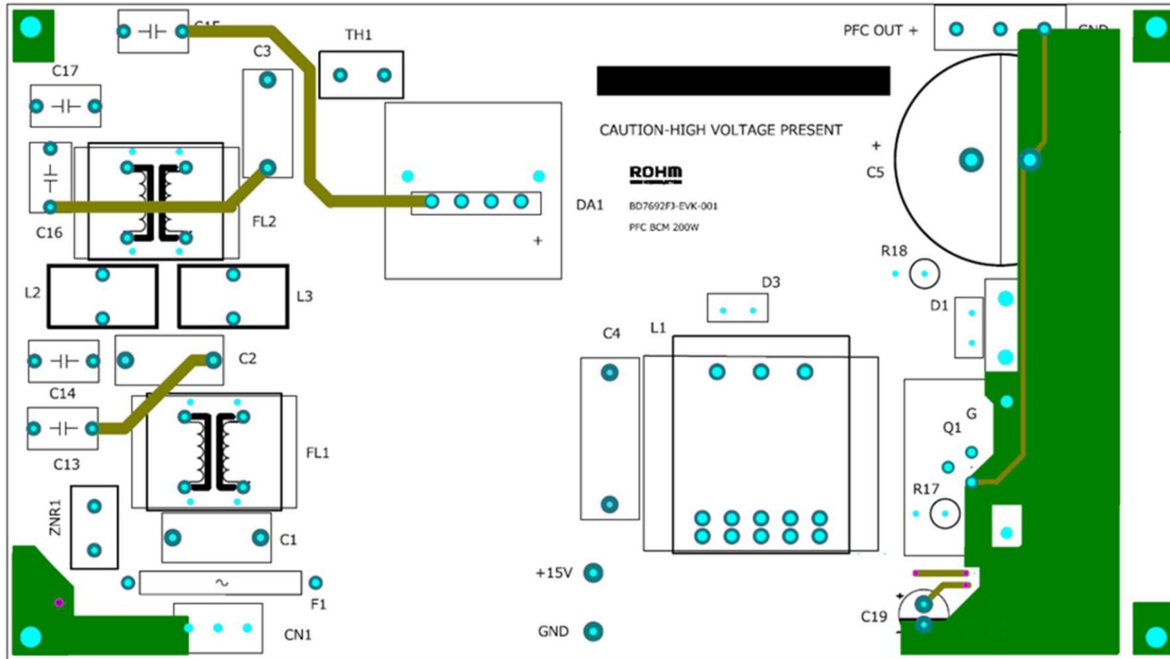
Top Layer
