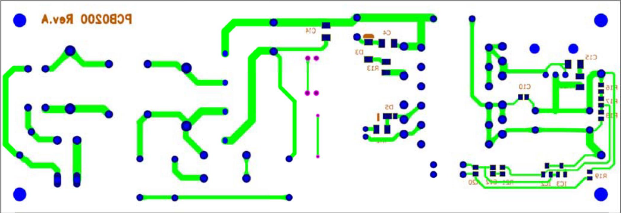
Bottom Layer
