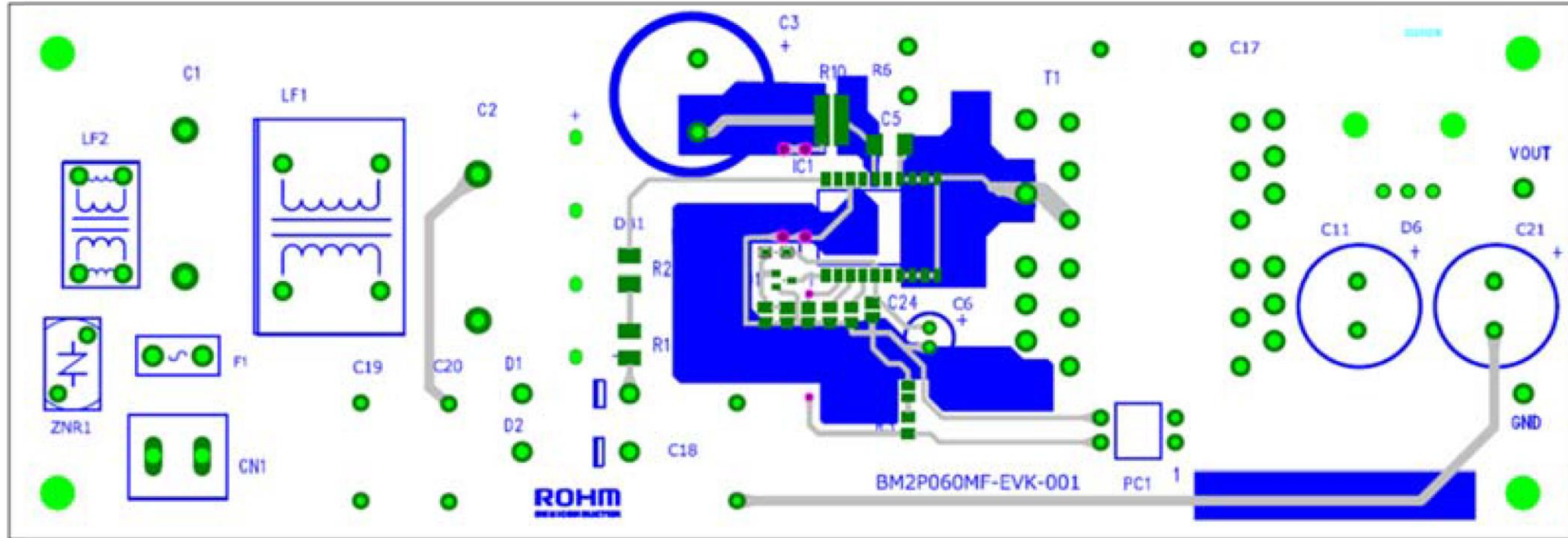
Top Layer
