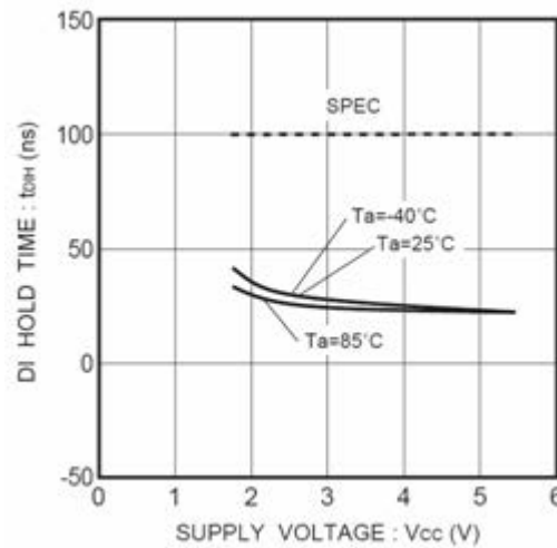
Figure 25. DI hold time tDIH
