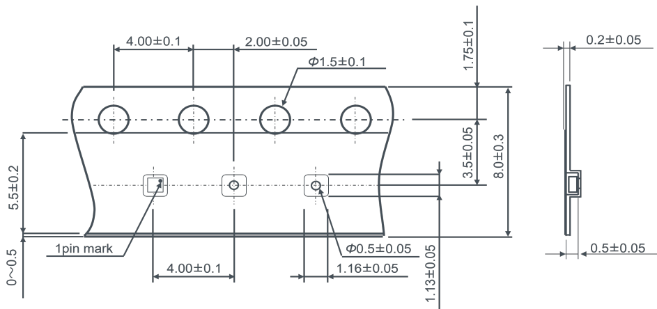
UNIT : mm
