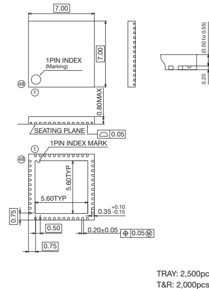
P-WQFN48-0707-0.50-63
