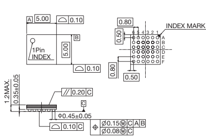
P-TFBGA36-0505-0.80-9
