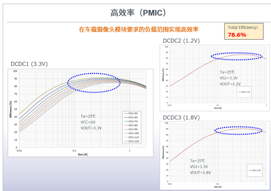
图 4 PMIC 的功率转换效率
