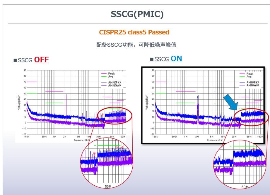
图 6 利用 PMIC 的 SSCG 功能实现的降噪效果
