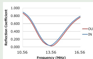
天线线圈谐振频率匹配特性
