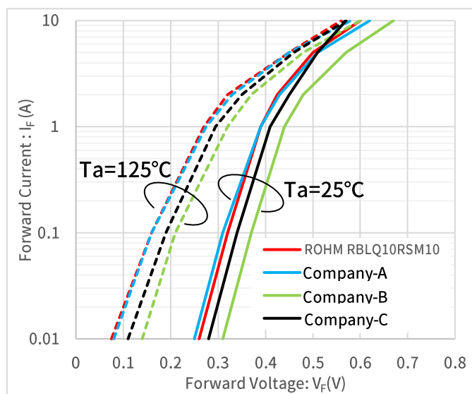
Figure 3. I_F - V_F 特性
